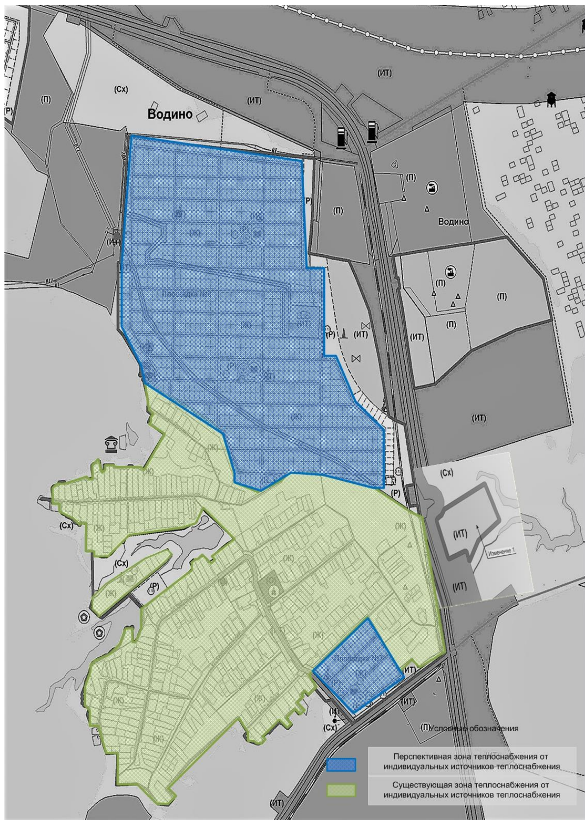
Рисунок 9 – Зоны действия существующих и перспективных источников тепловой энергии, находящихся в частной собственности жителей п. Водино.
