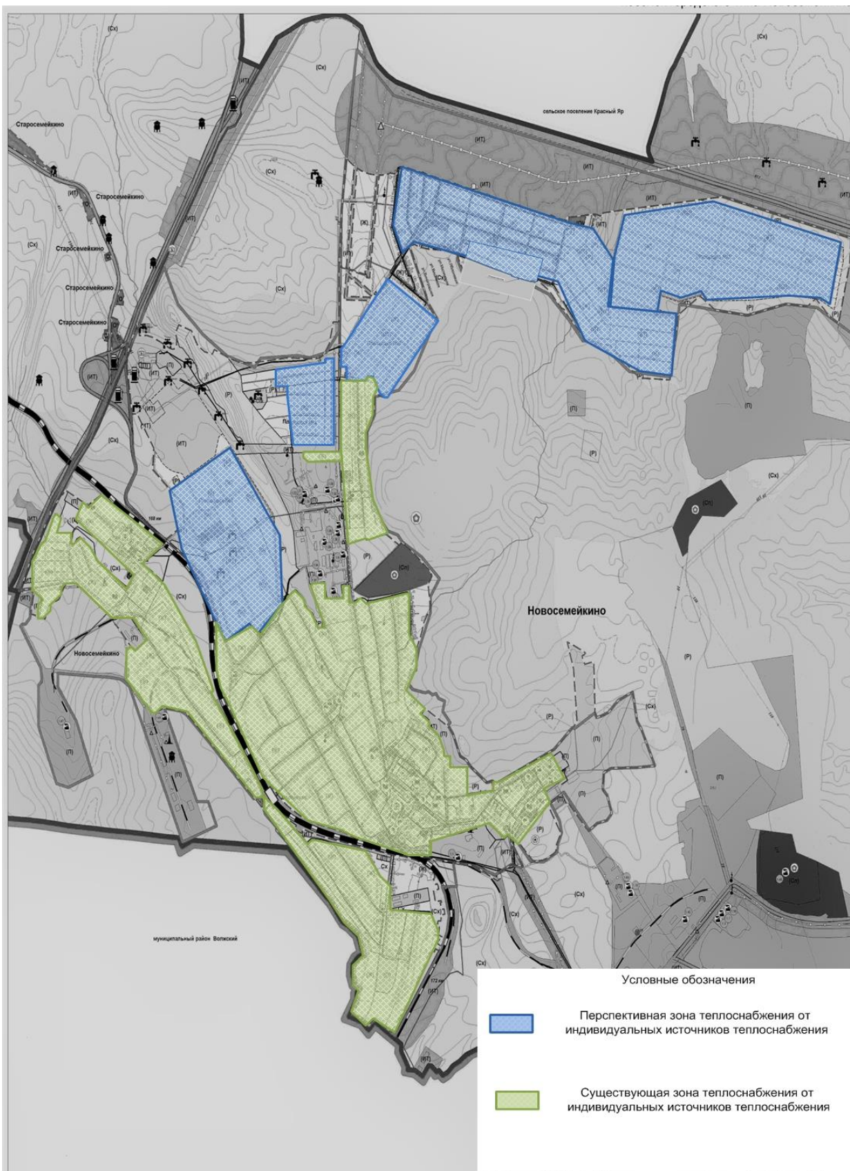
Рисунок 8 – Зоны действия существующих и перспективных источников тепловой энергии, находящихся в частной собственности жителей п.г.т. Новосе́мейкино
